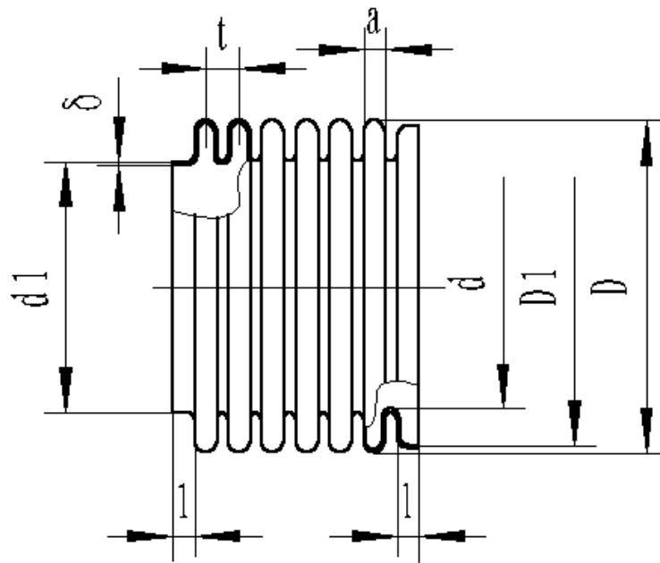
金属波纹管结构简图
